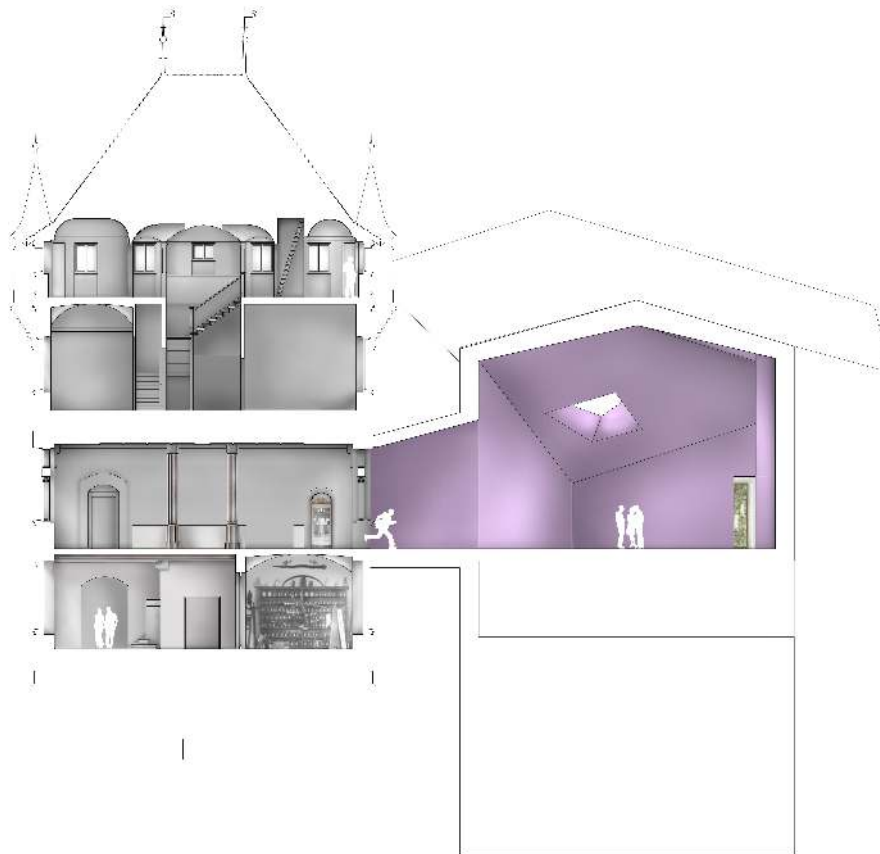
Alt und neu: Schnitt von Christ & Gantenbein.
